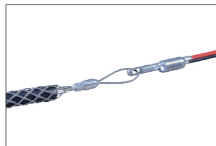
Cable malla de tracción – conector de rosca – RUNPOCAM – cable de alimentación con rosca RUNPOTEC RTG de Ø 6 mm. Para tirar de los cables inmediatamente.
