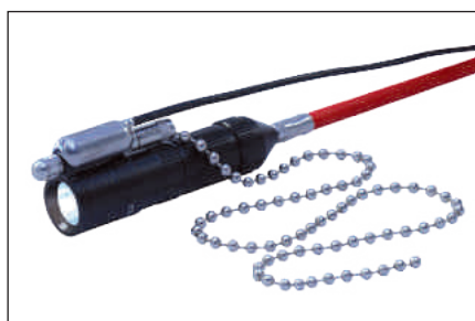
RUNPOCAM con cadena de bolas – lámpara LED recargable – RUNPOTEC cable de alimentación con rosca RTG de Ø 6 mm. Muy práctica cuando se combina con el imán.
