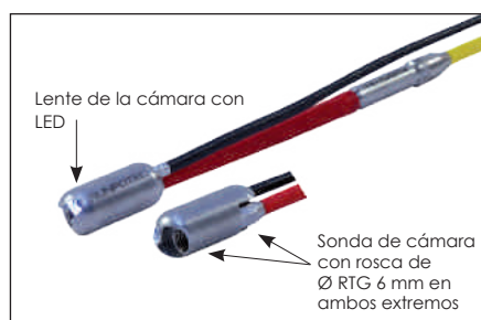
RUNPOCAM – RUNPOGLIDER con rosca frontal Para inspeccionar tuberías Ø 20 mm, Ø 25 mm y Ø 32 mm.
