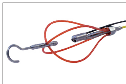
Gancho – deslizador funcional (dentro va la RUNPOCAM con base giratoria) – cable de alimentación con rosca RUNPOTEC RTG de Ø 6 mm. Para inspeccionar falsos techos.
