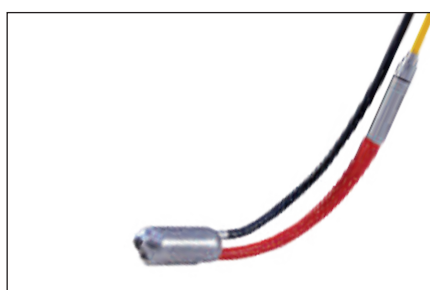
RUNPOCAM – RUNPOGLIDER con rosca frontal RUNPOTEC RTG de Ø 6 mm. Puede alcanzar radios más pequeños .
