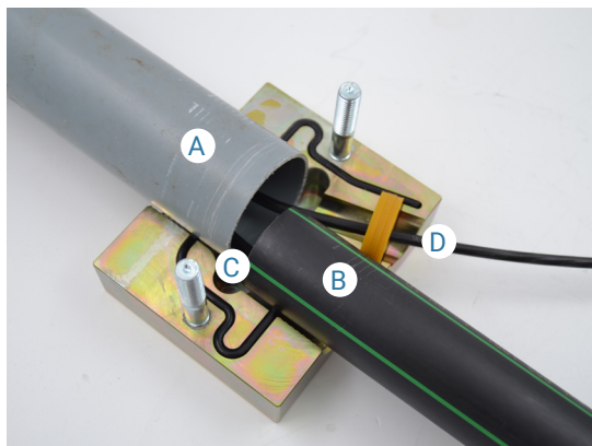
A) conducto existente de 50 mm, B) conducto de alimentación de 40 mm, C) Cable nuevo, D) Cable existente
