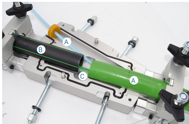
A) Cable o ducto de salida, B) Ducto de suministro, C) Cable nuevo
