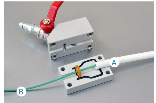
A) Microduct, B) Cable
