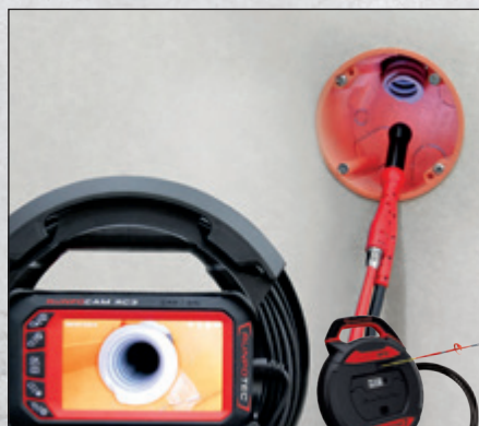
Inspección de tubos desde Ø 14 mm y más GF3 / RP1
